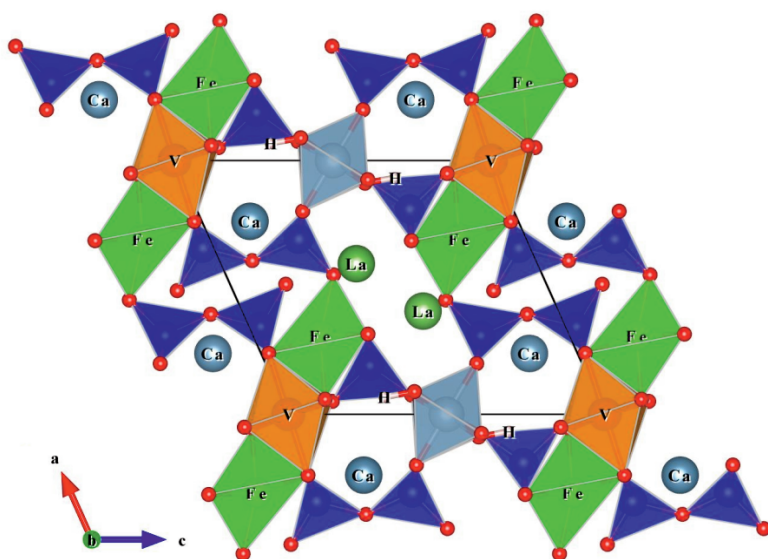
図1 ランタンバナジウム褐簾石の結晶構造図 緑色の球で示されるものがランタン、オレンジ色の八面体で示されるM1席にバナジウムが存在する。(VESTAで作成：Momma & Izumi 2011)
