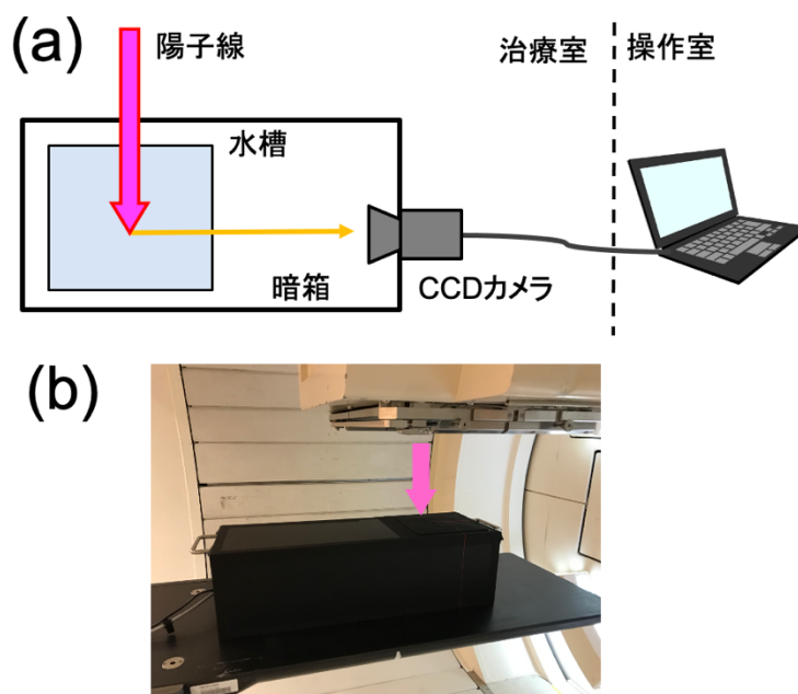
図 2. 測定装置の概念図(a)と写真 (b)
