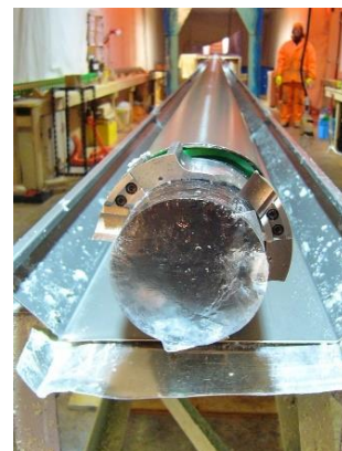
図1：(左) 東南極の主な掘削地点。 (右) ドームふじ基地で掘削されたアイスコア。
